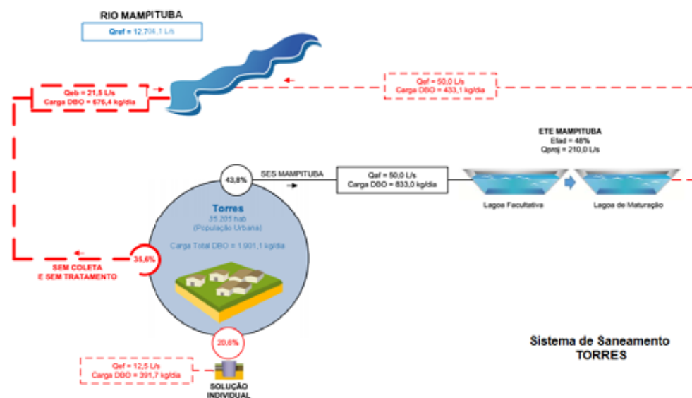
Esquemática do Sistema de Saneamento atual em Torres (fonte: ANA)
